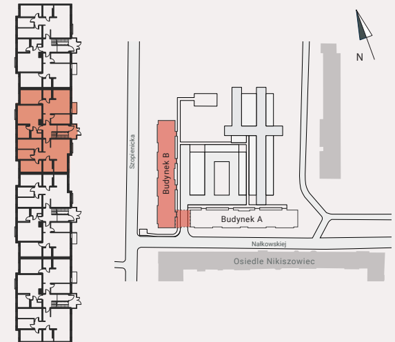
Budynek B - parter - segment B3
