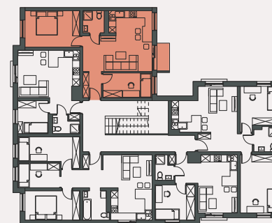
Budynek B - 3 piętro - segment B1
